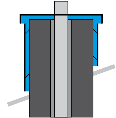
Prinzip der Schornsteinverkleidung
